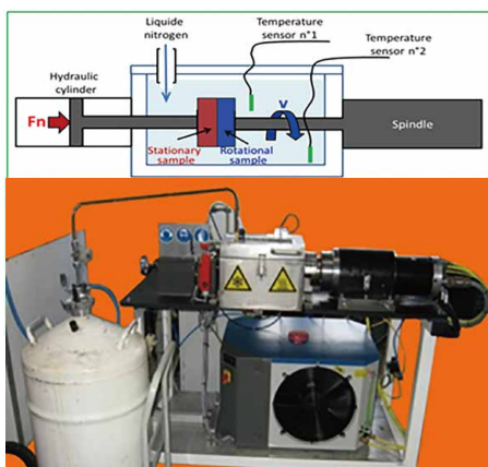
High speed/Cryogenic Tribometer ~ 20000 rpm, -200/350°C 高速 / 極低温トライボメータ
